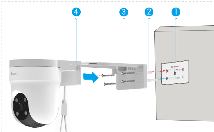
그림 2 벽 장착
