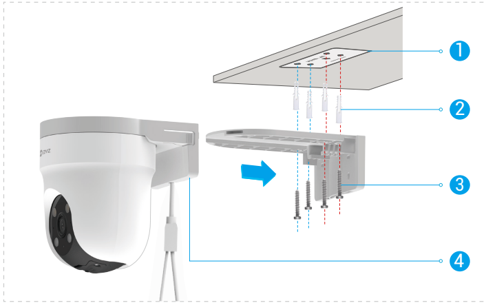
그림 1 천장 장착
